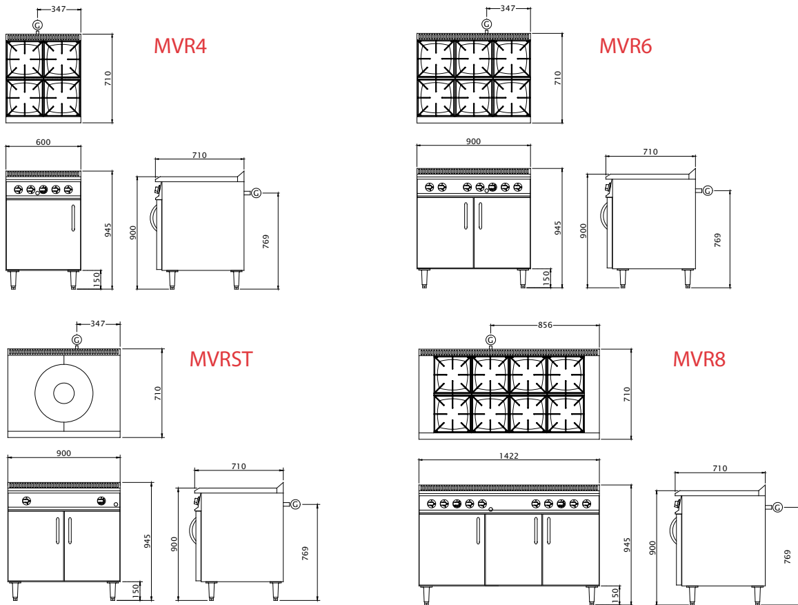
DIMENSIONS
